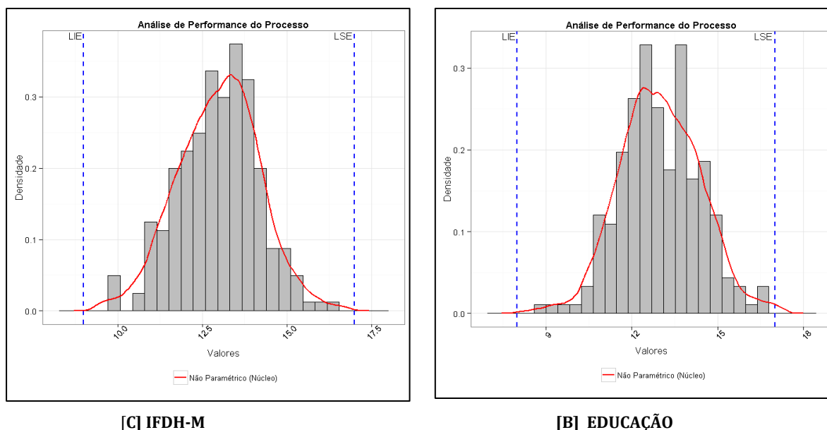
Figura 2: Histograma e funções de densidade (Kernel Density) dos Índices: Fonte: Elaboração Própria.
